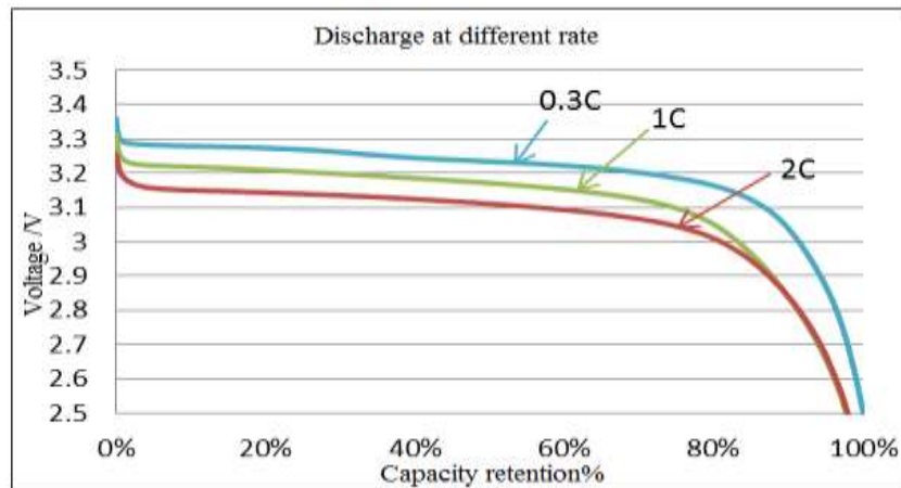
图 1. SE200 常温放电曲线
